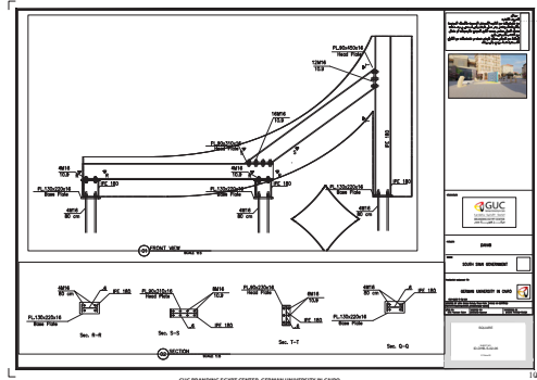
الرسم الانشائي لحروف كلمة دهب
