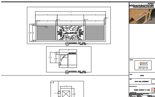
الرسم المعماري لمظلات المحلات
