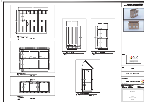
الرسم المعماري لسلات القمامة
